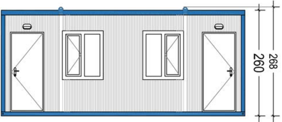
წინა ხედი FRONT VIEW
